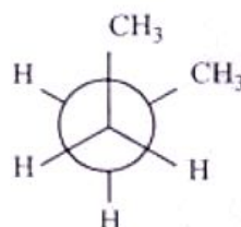
Gauche
