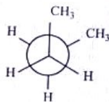
Gauche
